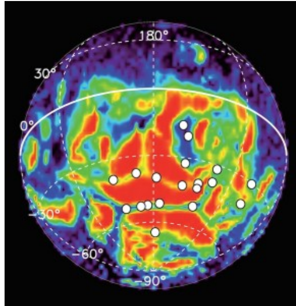
Carte de distribution des aurores discrètes (cercles blancs) recensées par le Pr Gérard dans l'hémisphère sud de Mars. Le paléomagnétisme apparaît en fond de carte. © ULg, ESA (Cliquer pour agrandir)
