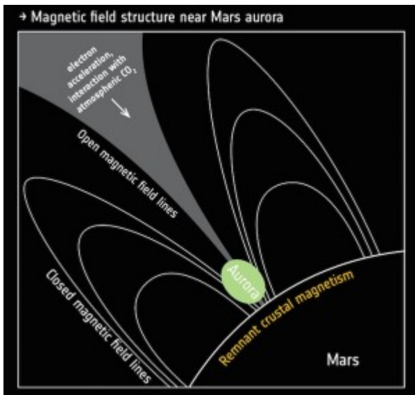
Mars Express: mécanisme des aurores discrètes. © ESA
